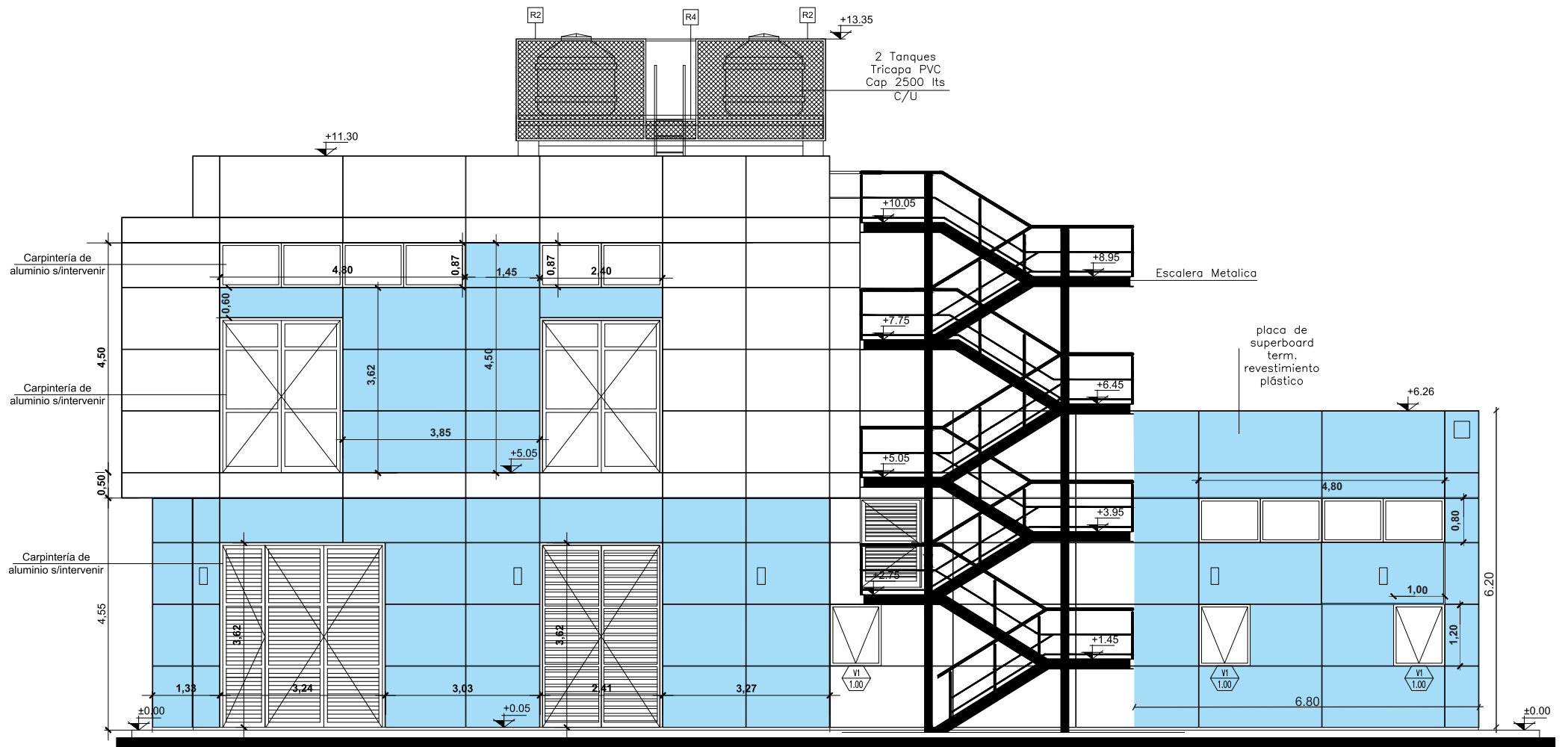
FACHADA ESTE sobre calle Valparaiso
