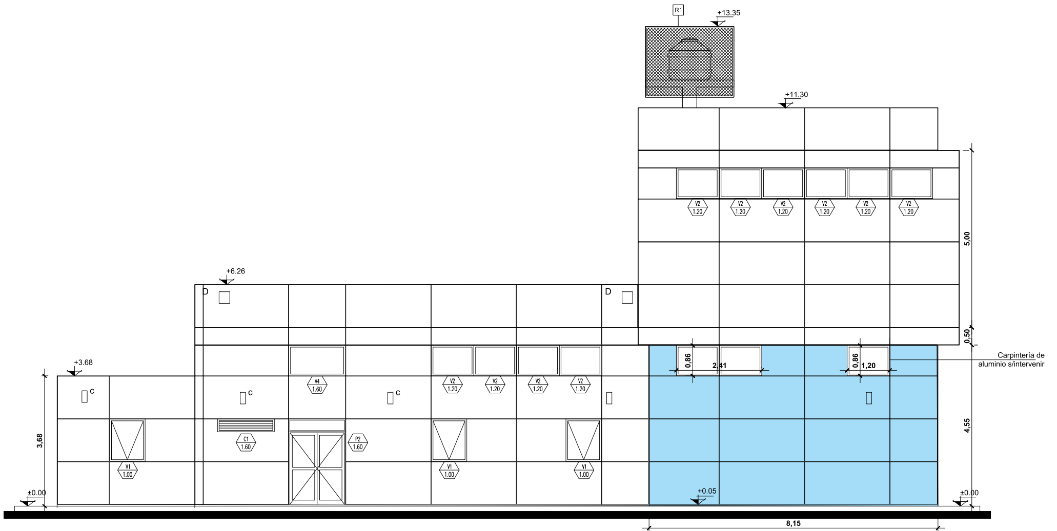
FACHADA SUR sobre calle Filloy
